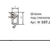
Штапик под стеклопакет 24 мм Арт. № 107.210
