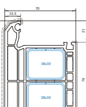
Импост 118 мм Арт. № 102.202 усилитель арт. № 113.271 / 2 шт. усилитель для ответных частей входной двери, арт. № 113.302
