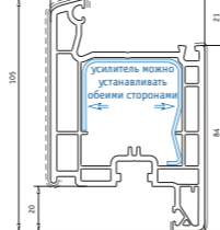
Створка 105 мм, внешнего открывания Арт. № 103.247 усилитель арт. № 113.270 усилитель алюминиевый арт. № 115.003
