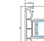
Импост 85 мм Арт. № 102.214 сталь: 30x30/113.025
